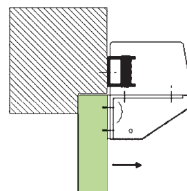
Montage extérieur inversé sur équerre
