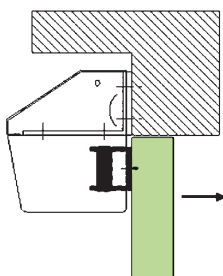
Montage sous équerre porte affleurante
